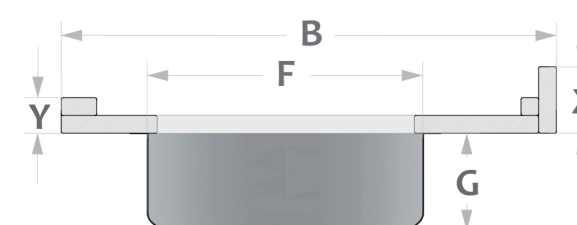
CORTE TRANSVERSAL
